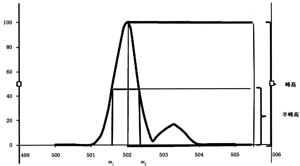
图 A.1 人工测量计算 W_{1/2} 的模拟图
